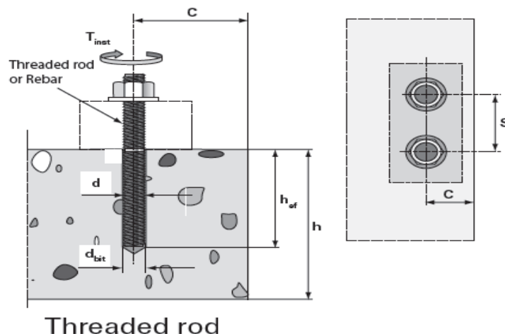
FIGURE 1—INSTALLATION PARAMETERS
